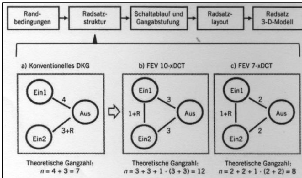
Abbildung 1: Darstellung einer Radsatzsynthese sowie Radsatzstrukturen Quelle: Hellenbroich, G.; Ruschhaupt, J.; Duidam, C. (2012), S. 962
